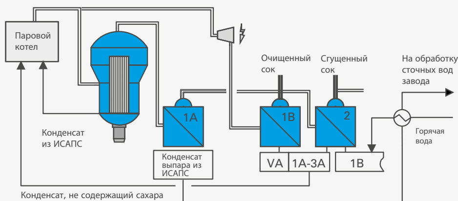
Выпарная установка с испарительным сушильным аппаратом с псевдооживленным слоем
