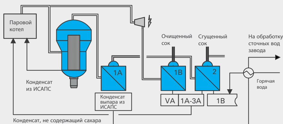
Выпарная установка с испарительным сушильным аппаратом с псевдоожиженным слоем
